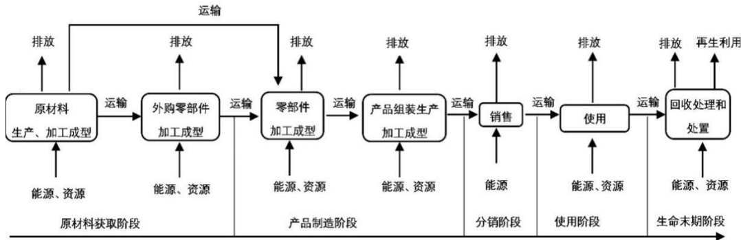
图1 洗衣机产品碳足迹量化的系统边界示例
